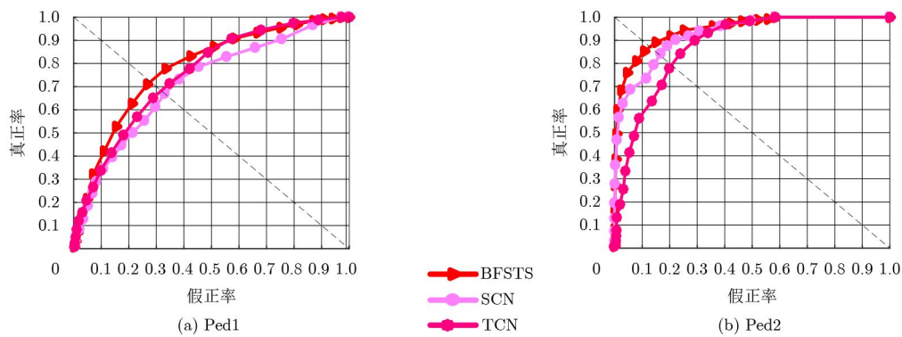
图7 UCSD Ped1和Ped2数据库基于规则分数的ROC曲线
