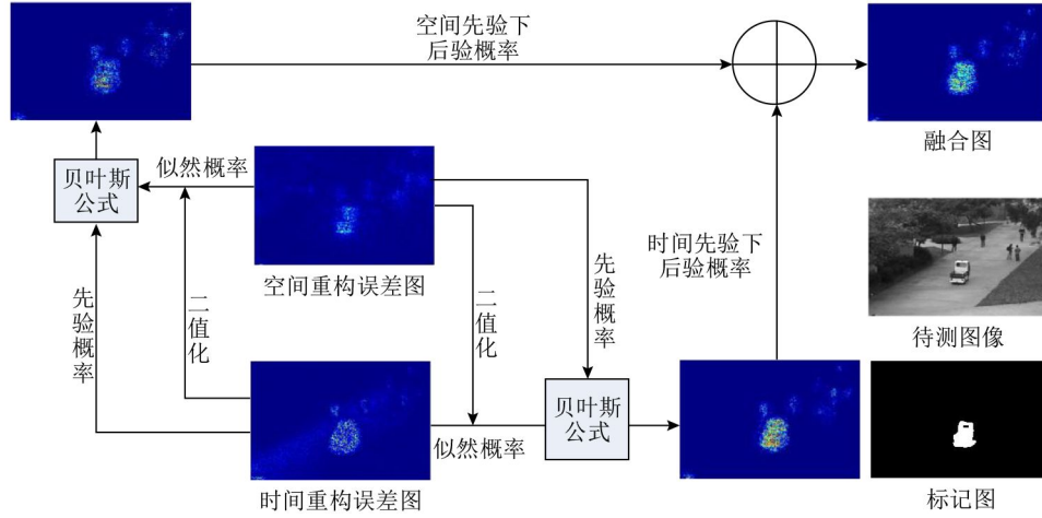
图4 基于贝叶斯的时空流融合图
