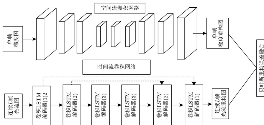
图1 基于贝叶斯融合的空-时流异常行为检测整体框架
