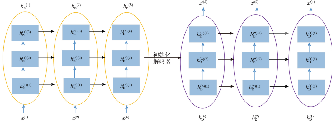
图3 Conv-LSTM编码-解码过程
