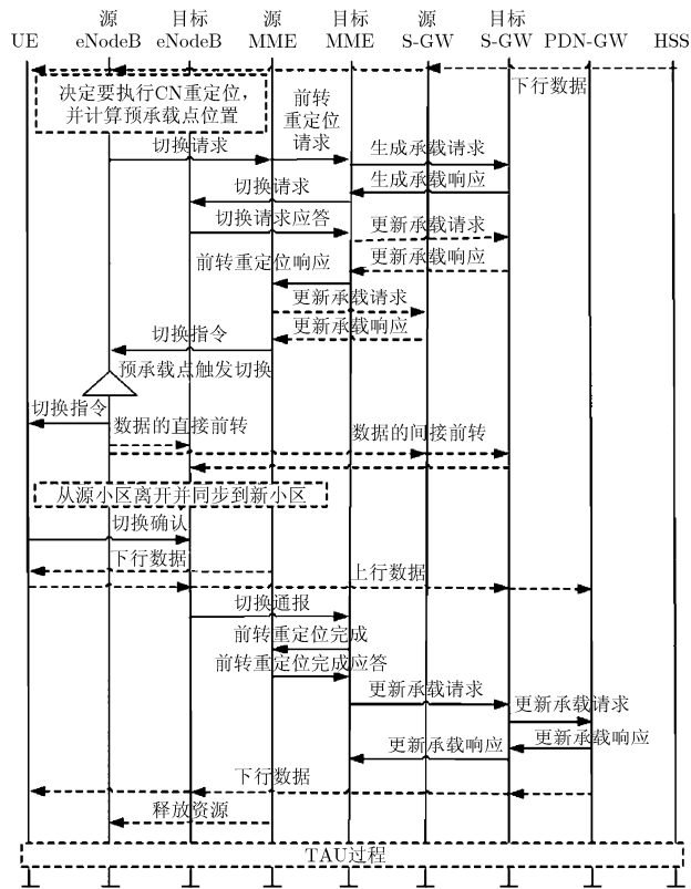
图 3 基于速度触发的提前切换算法信令流程(S1)
