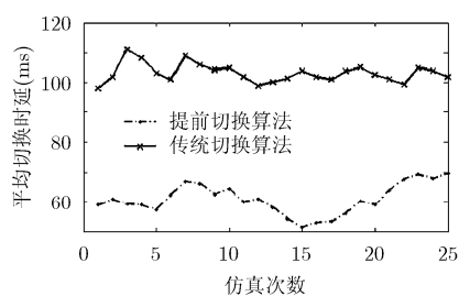
图4 两种切换算法系统时延对比图
