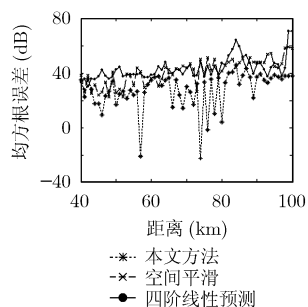
图 4 不同距离目标高度均方根误差对比图
