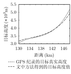
图 5 某米波雷达实测数据处理结果
