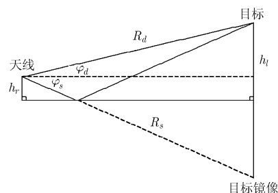
图 1 接收天线模型
