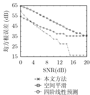
图 3 不同信噪比目标高度均方根误差对比图
