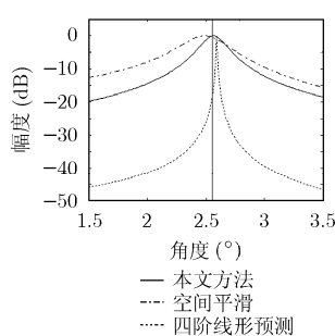
图 2 3 种方法俯仰角测量结果
