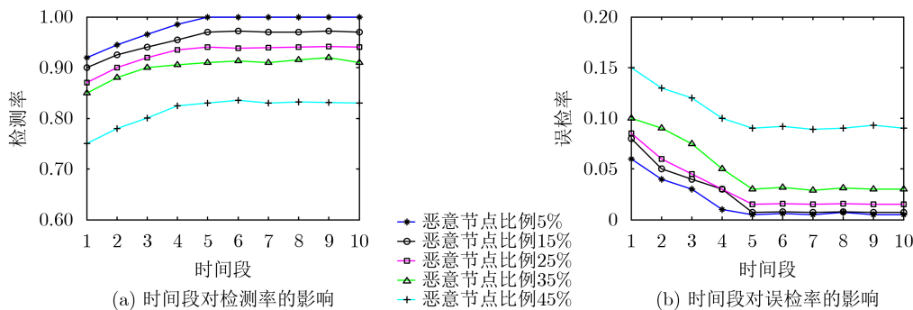
图3 时间段对检测率和误检率的影响
