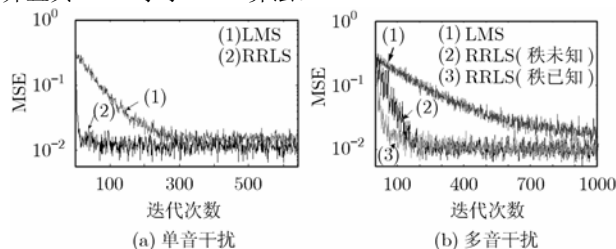
图 2 RRLS 算法收敛特性曲线
