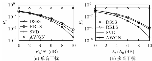
图 3 接收机误码率曲线
