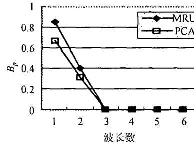
图 3 阻塞率-波长数曲线
