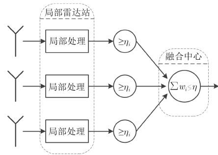
图1 CDDF算法流程示意图
