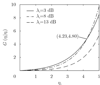
图6 不同输出信杂噪比条件下 G(\eta_i)
