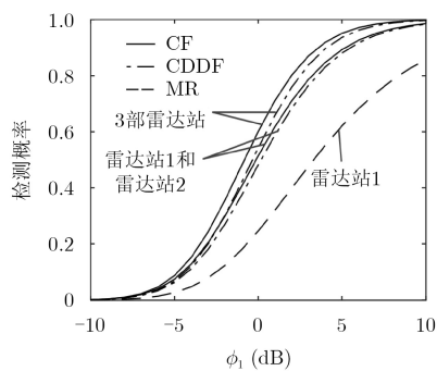
图5 CF和CDDF融合检测性能
