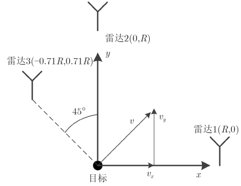
图2 多基地雷达系统的位置信息
