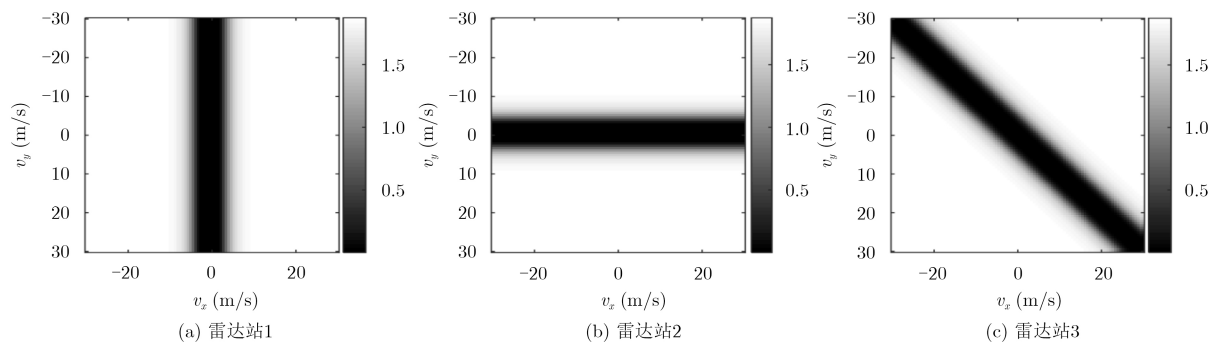
图4 局部雷达站的偏移系数同速度分量的关系
