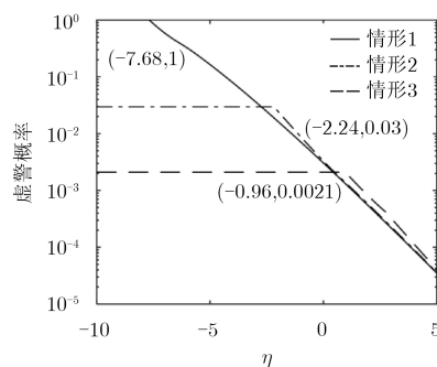
图7 全局门限同虚警概率之间的关系
