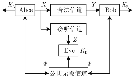
图3 信道型密钥生成模型
