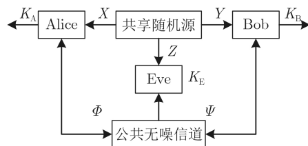
图2 源型密钥生成模型
