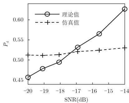
图8 对偶序列跳频信号的随机共振检测性能随SNR变化情况
