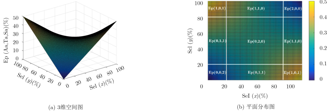
图3 N_{OB} = 2 时概率期望 E_{Pr}(Aa, Ta, Sa) 的分布图
