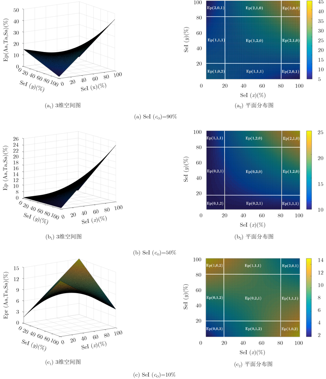
图4 N_{OB}=3 时概率期望 E_{Pr}(Aa, Ta, Sa) 的分布图
