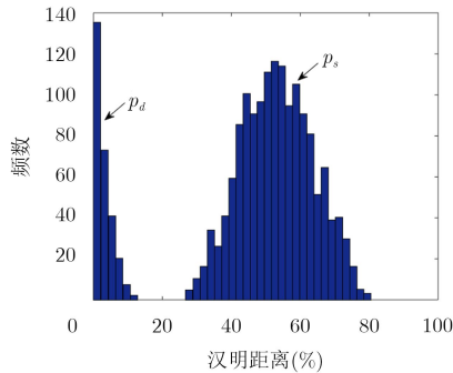
图7 控制型PUF响应的汉明距离频率分布图
