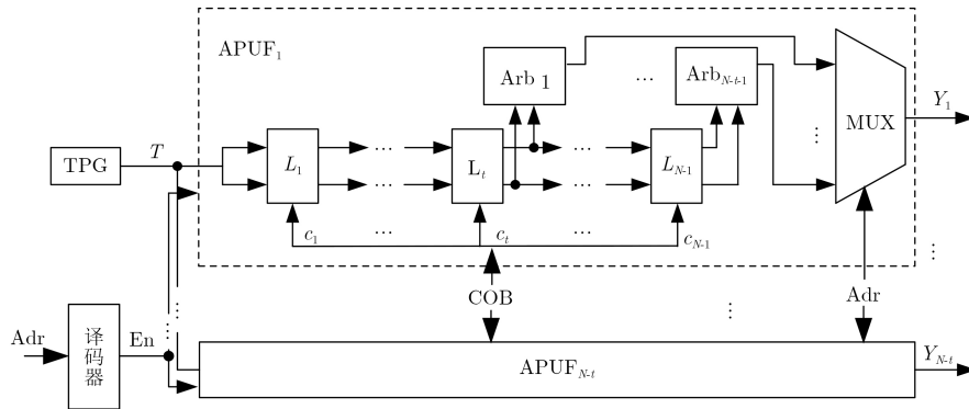
图6 基于APUF的混淆值产生模块
