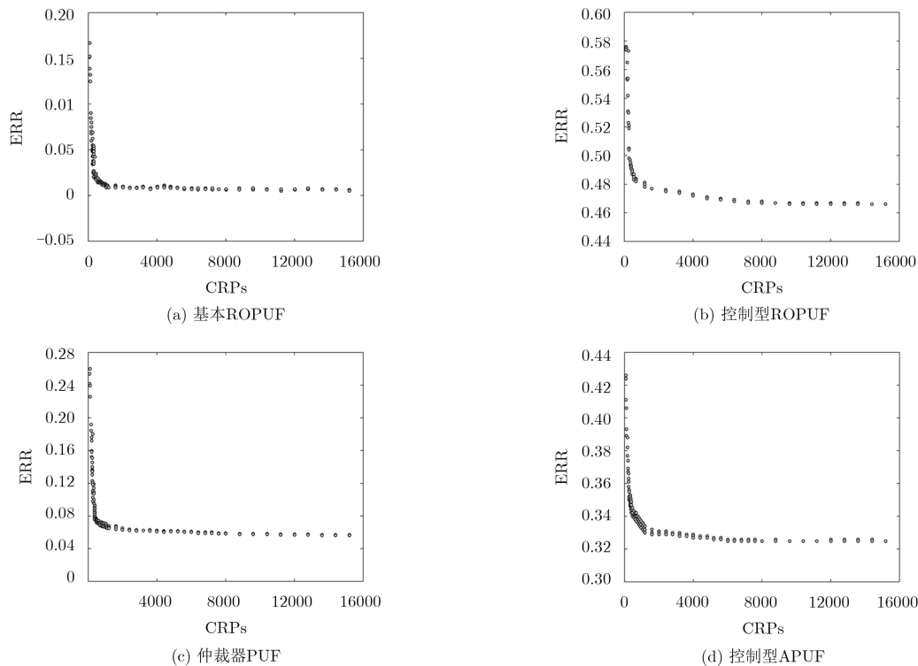
图8 不同PUF结构的建模攻击结果
