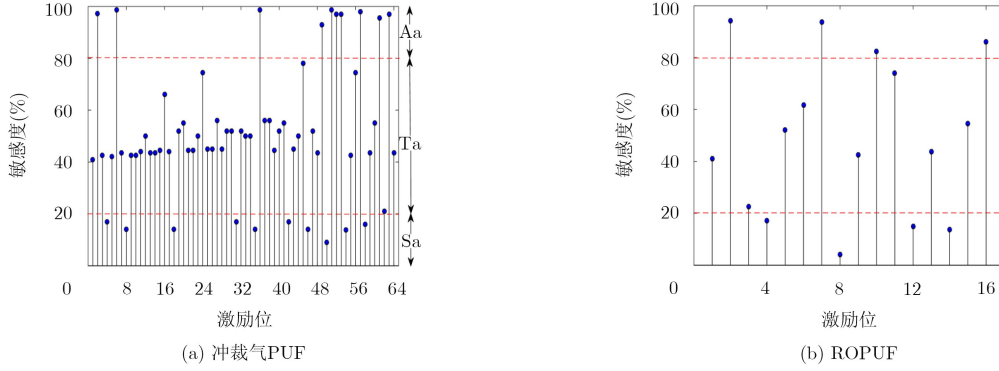
图2 敏感度测量结果
