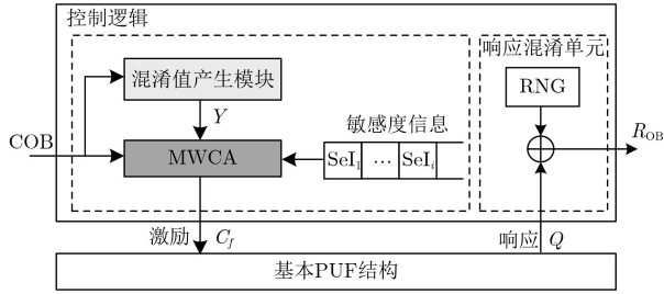
图5 基于敏感度混淆机制的控制型PUF架构
