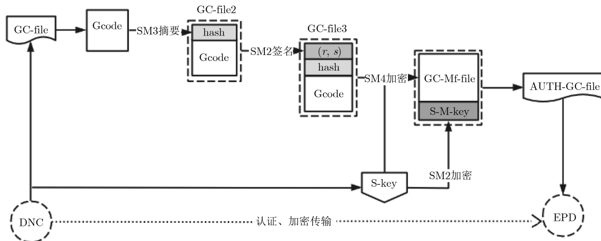
图1 NCS网络AUTH-VRF模型安全认证流程
