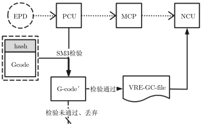
图 2 NCS网络AUTH-VRF模型安全验证流程
