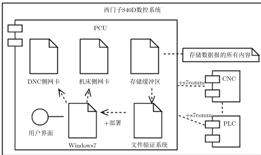
图 5 内层防护装置部署概况
