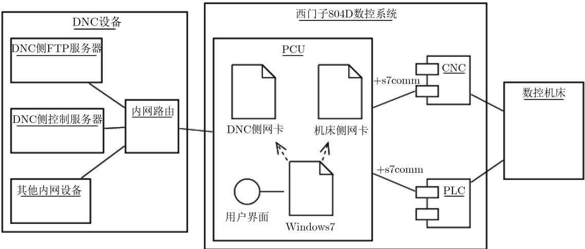
图 3 AUTH-VRF模型实现场景部署
