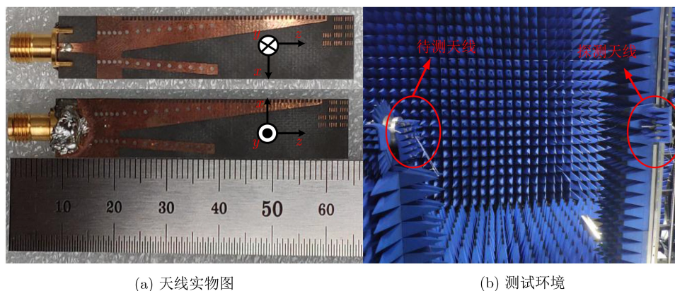
图7 天线测试
