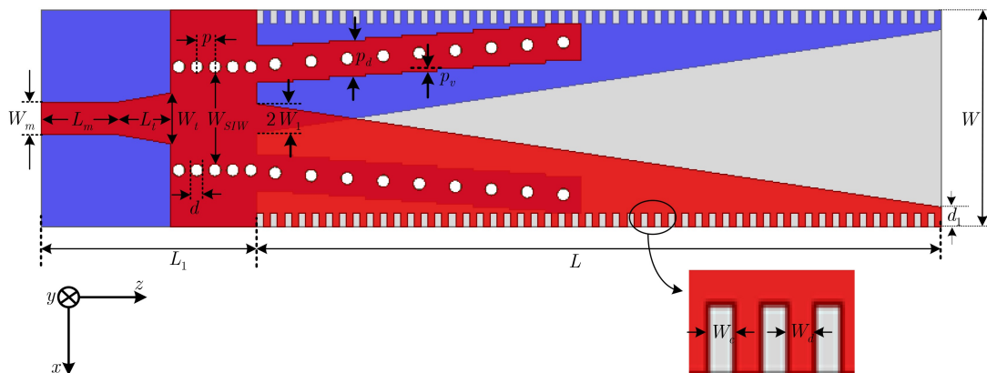
图1 基于SIW馈电的对距直线渐变缝隙天线 W
