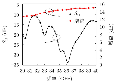
图2 ALTSA结构 S_{11} 及增益曲线
