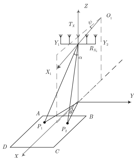
(a) FLMC-SAR几何模型
