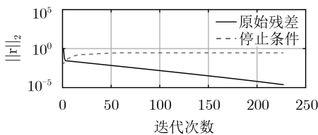
(a) 原始残差随迭代次数变化
