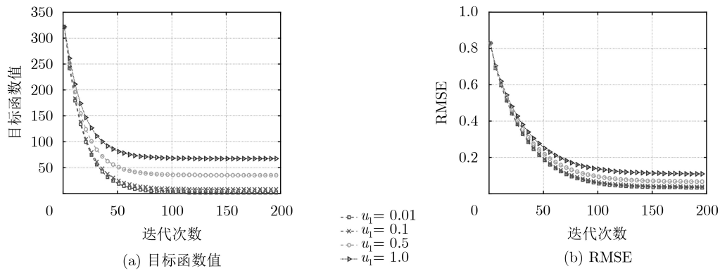
图 8 参数 u_1 对算法性能的影响
