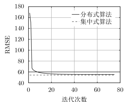
图 12 RMSE随迭代次数变化
