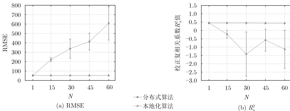
图 13 分布式算法与本地化算法之间的性能比较
