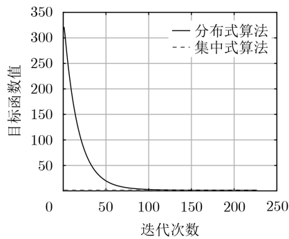
图2 目标函数值随迭代次数变化
