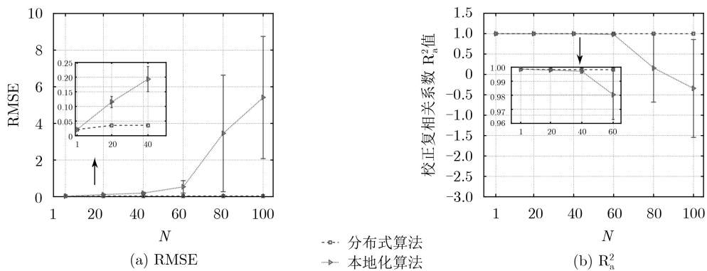
图 10 分布式算法与本地化算法之间的性能比较
