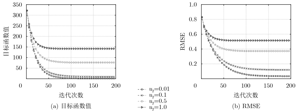
图 9 参数 u_2 对算法性能的影响
