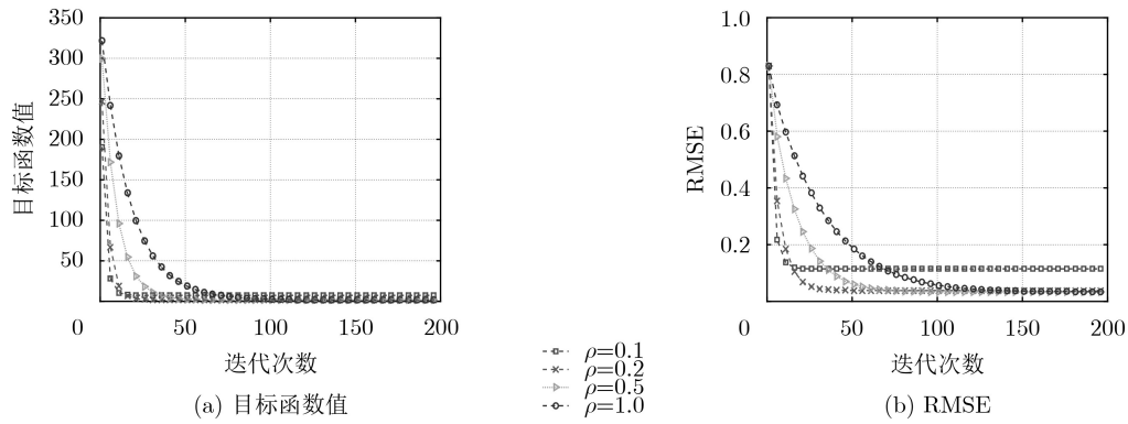
图 7 参数 \rho 对算法性能的影响
