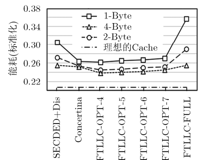
图8 不同的末级缓存在不同粒度下的能耗开销
