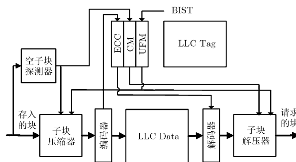
图 1 FTLLC 设计结构
