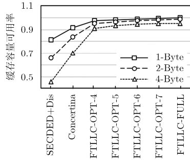
图4 不同的末级缓存在不同粒度下的容量可用率
