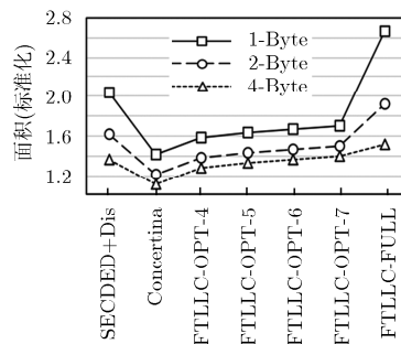
图7 不同的末级缓存在不同粒度下的面积开销
