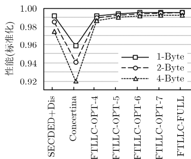
图6 不同的末级缓存在不同粒度下的性能
