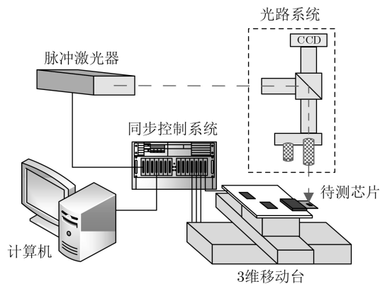
图3 实验平台
