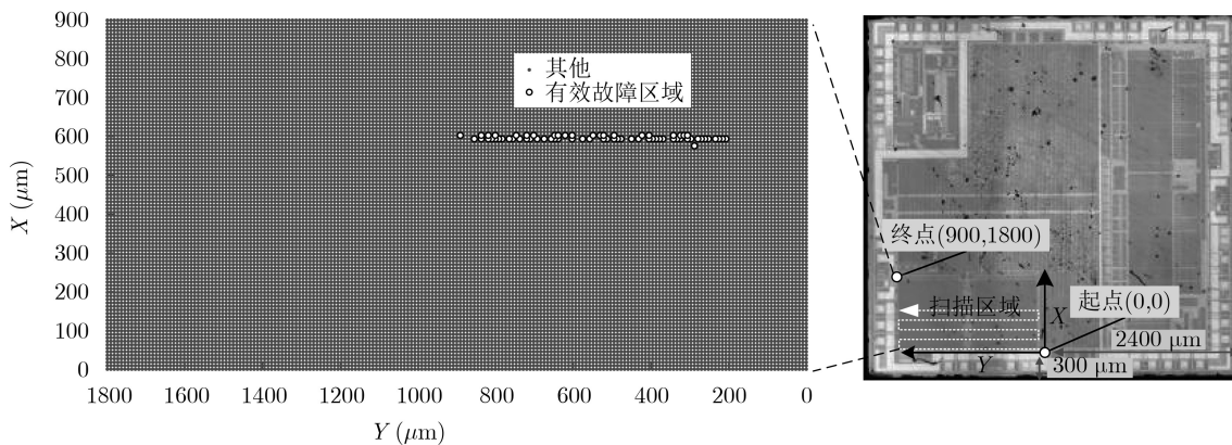
图6 差分故障攻击的有效区域
