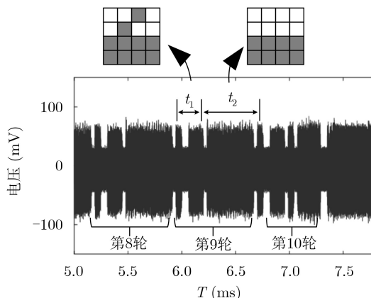
图7 后3轮功耗及攻击子密钥的有效时间段
