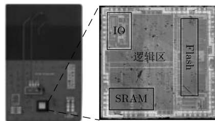
图4 ATMEGA163L型微控制器及背部的版图
