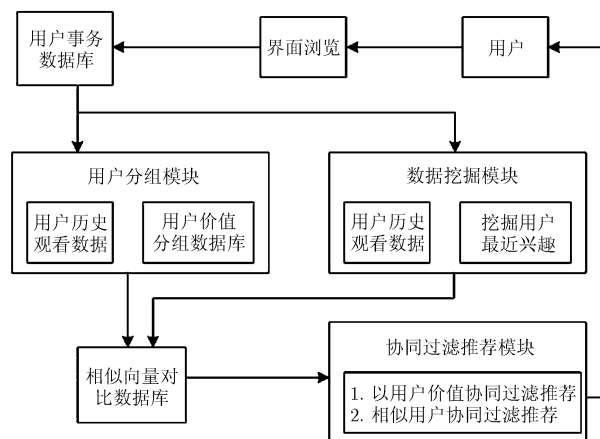
图1 基于用户行为分析的视频推荐流程图
