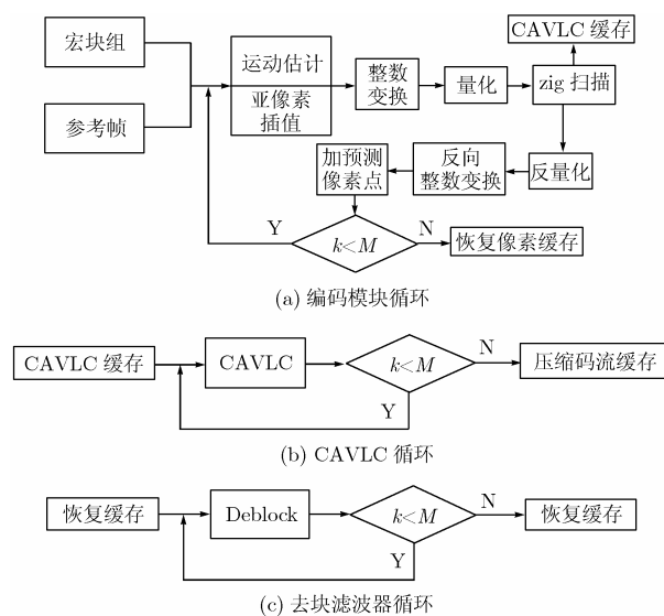
图6 循环模块
