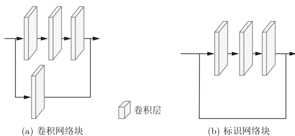
图2 两种残差网络块的结构图
