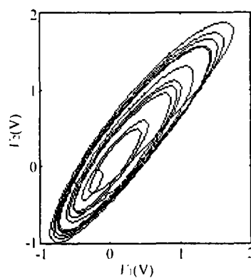
图 8 采用三段线性 VCVS 时的混沌吸引子
