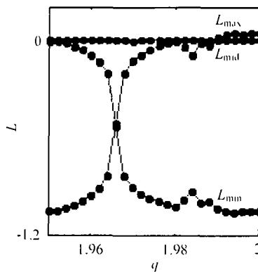
图 4 系统的三个李雅普诺夫指数 ( L_{\max}, L_{\text{mid}}, L_{\min} ) 随 q 的增加而发生变化
