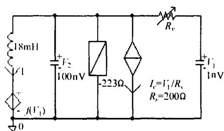
图 5 实现混沌发生器的电路结构
