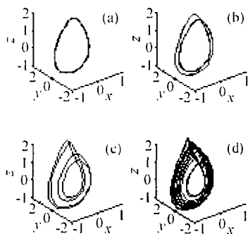
图 1 倍周期分岔导致混沌
