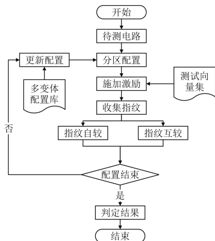
图7 算法检测流程示意图
