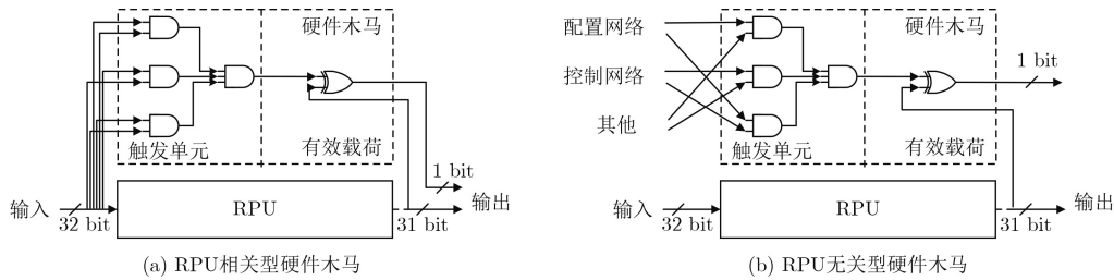
图2 不同触发信号的硬件木马示意
