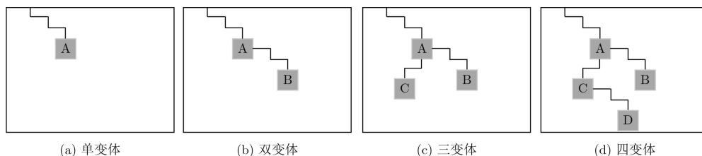
图5 子任务不同变体执行实例
