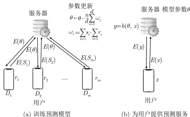
图4 安全数据聚合协议
