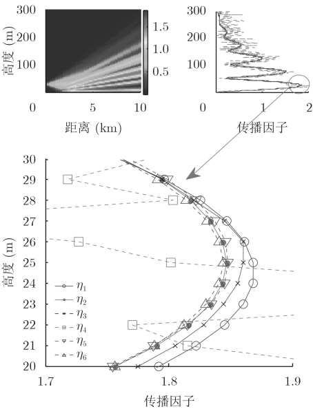
图2 光滑海面仿真结果
