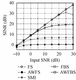
图 4 阵列输出 SINR 随 SNR 的变化
