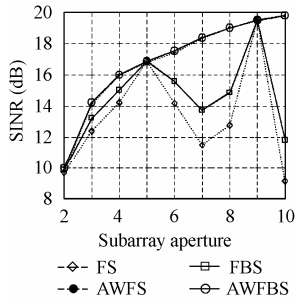
图 3 阵列输出 SINR 随子阵孔径的变化
