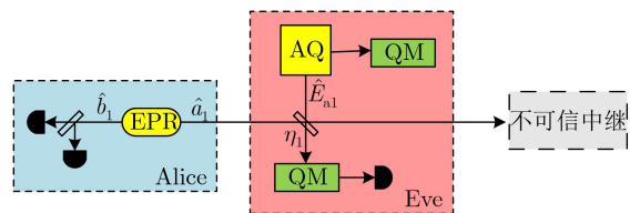
(b) 等价纠缠模型时攻击方案图
