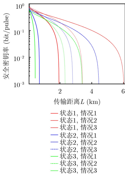
图4 4用户参与QSS协议安全密钥率和传输距离的关系
