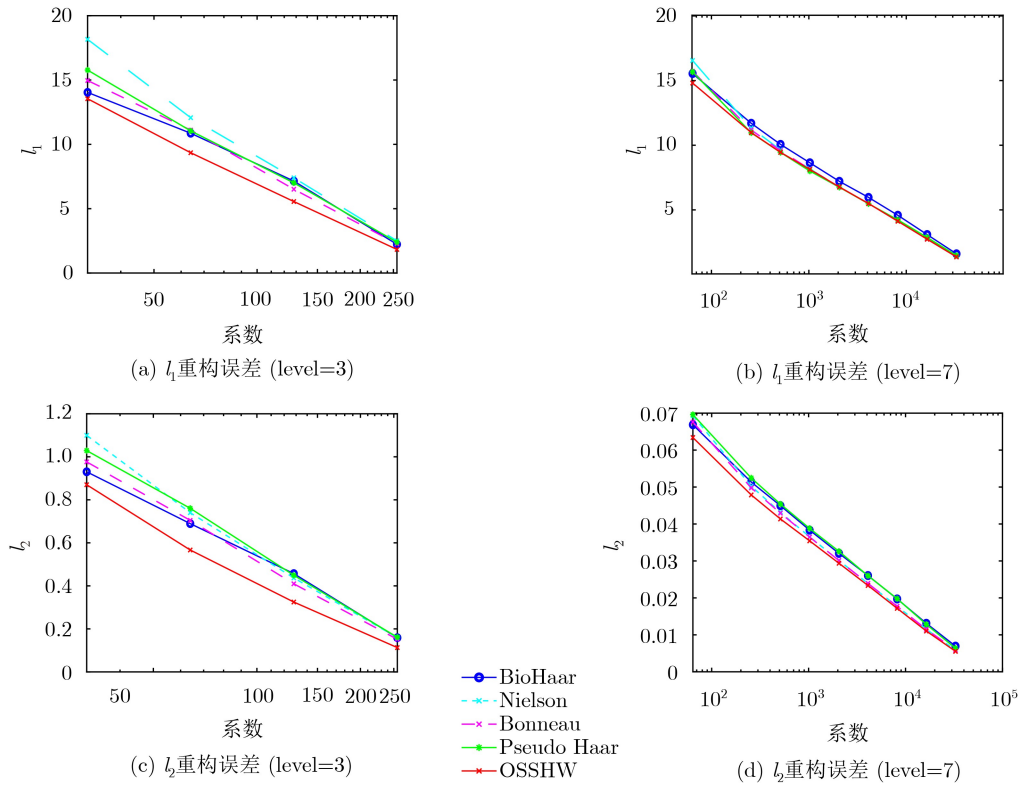
图4 虹膜信号重构误差
