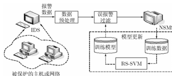
图 1 基于 RS-SVM 的误报警过滤系统的框架
