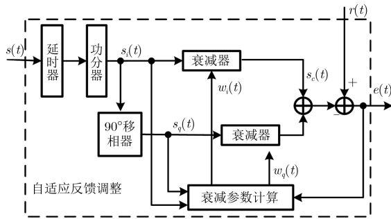
图1 单发单收射频干扰对消基本原理图
