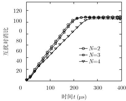
图4 同车发送电台数目 N 对应的MICR收敛曲线
