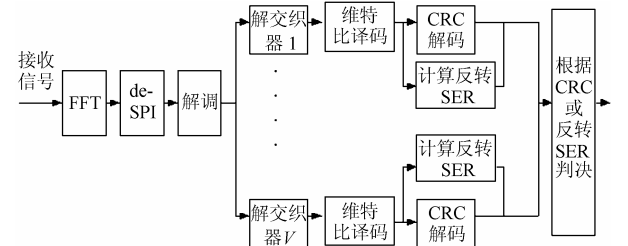
图2 NSI-IPR-OFDM 系统接收端框图
