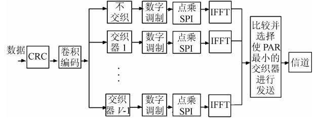
图1 NSI-IPR-OFDM 系统发送端框图
