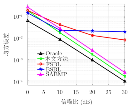
图2 信道估计均方误差随信噪比变化曲线图
