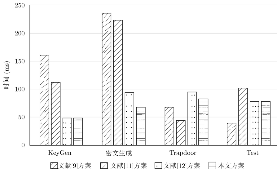
图 2 计算量对比
