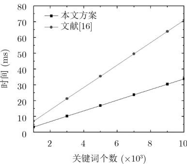
图 2 加密时间
