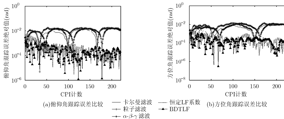
图7 角度跟踪环路性能比较
