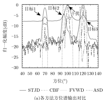
(a) 各方法方位谱输出对比
