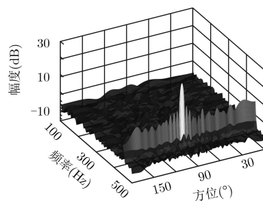
(b) STJD方法的方位频率域波束输出
