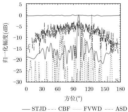
(a) 各方法方位谱输出对比
