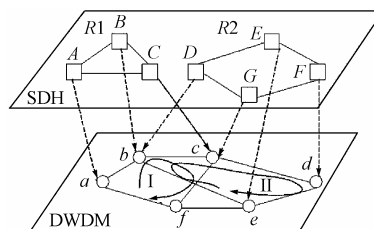
图4 SDH over DWDM 网络结构
