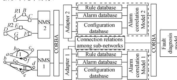
图5 分布式告警相关性模型的实现框架
