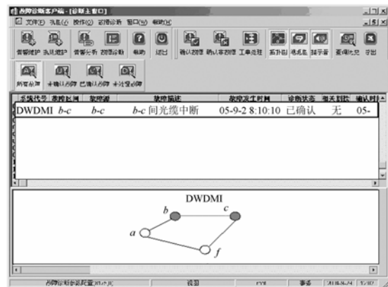
图 7 故障诊断结果
