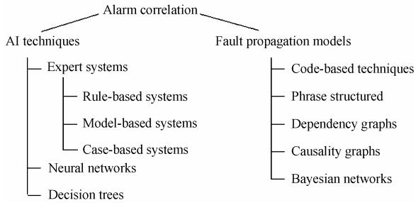
图 1 告警相关性分析模型
