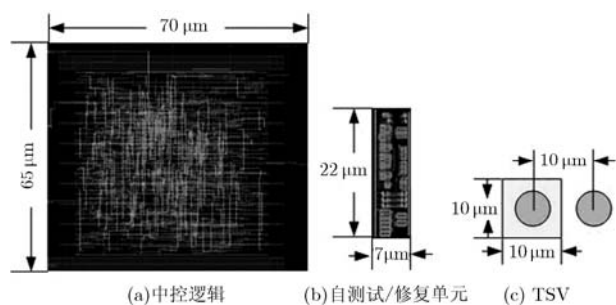
图9 版图
