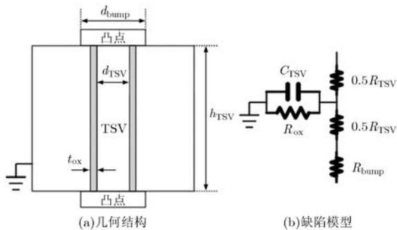
图 1 TSV 缺陷模型
