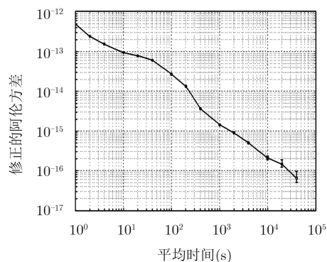
图9 光纤双向频率传递稳定度结果
