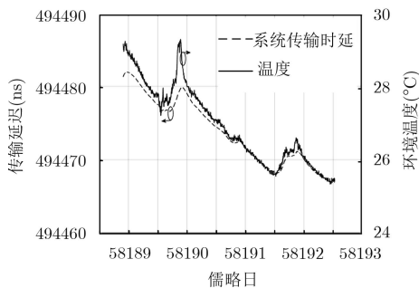
图3 时延测量结果与温度变化曲线
