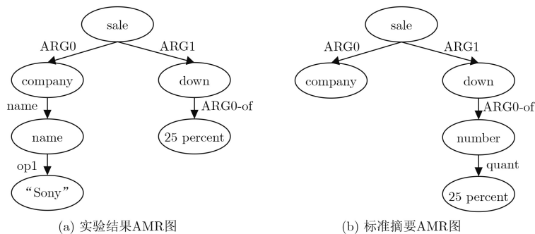
图4 实验结果AMR图与标准摘要AMR图的对比
