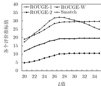
图5 L 值对摘要质量各指标的影响
