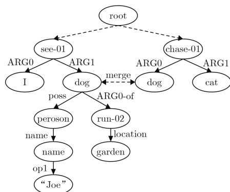
图3 AMR图合并生成AMR总图示意图
