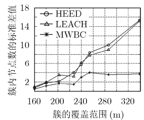
图2 簇内节点数的标准差与簇半径的关系
