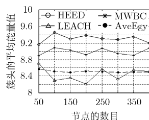
图7 簇头的平均能量与网络规模的关系
