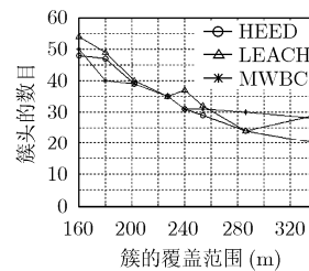
图1 簇的数目与簇半径的关系
