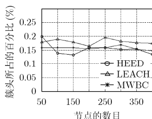
图4 簇的数目与网络规模的关系
