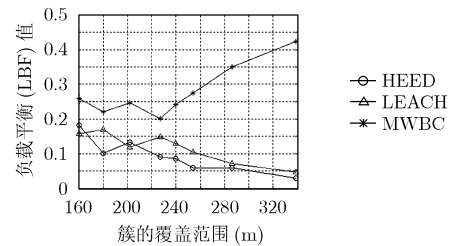
图3 网络的 LBF 值与簇半径的关系
