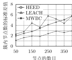
图5 簇内节点数的标准差与网络规模的关系
