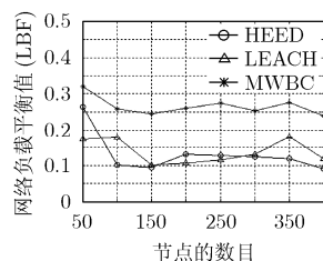
图6 网络的LBF值与网络规模的关系
