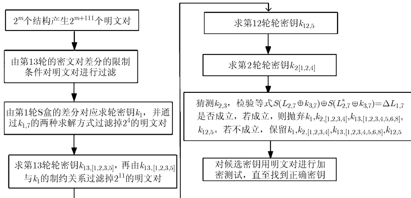
图 2 13 轮 MIBS-80 的不可能差分攻击流程图
