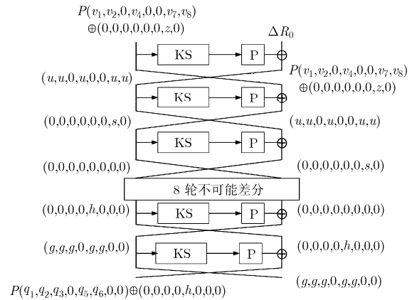
图 1 13 轮 MIBS-80 的不可能差分攻击
