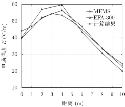
图 9 10 kV输电线路下电场测试与计算曲线
