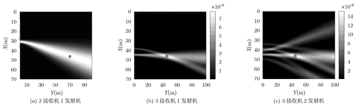
图3 不同接收机发射机的点目标仿真成像结果
