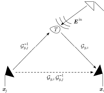
图1 无源回波模型构造原理示意图
