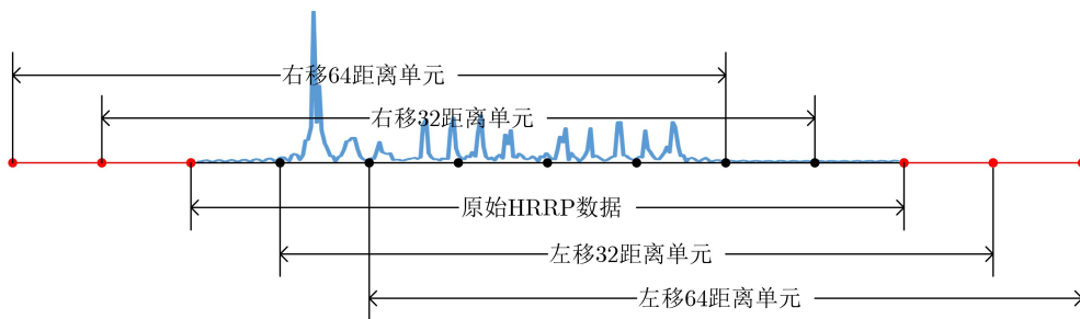
图6 HRRP数据平移截取示意图
