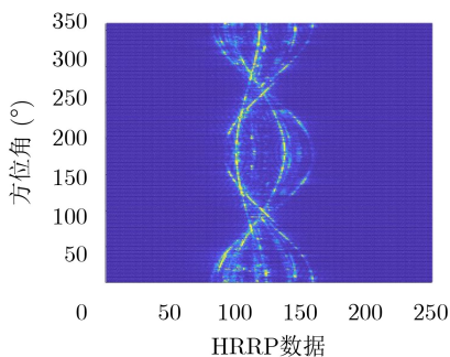
(b) 幅值归一化后的HRRP图
