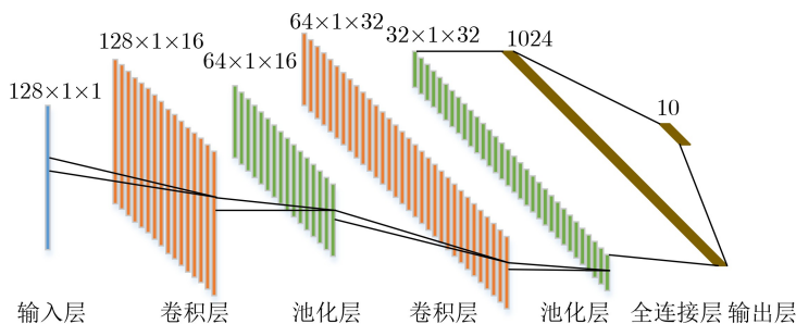
图1 针对HRRP的CNN结构示意图
