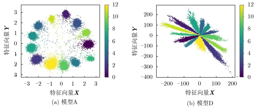
图7 信噪比为15 dB时不同模型的特征可视化图
