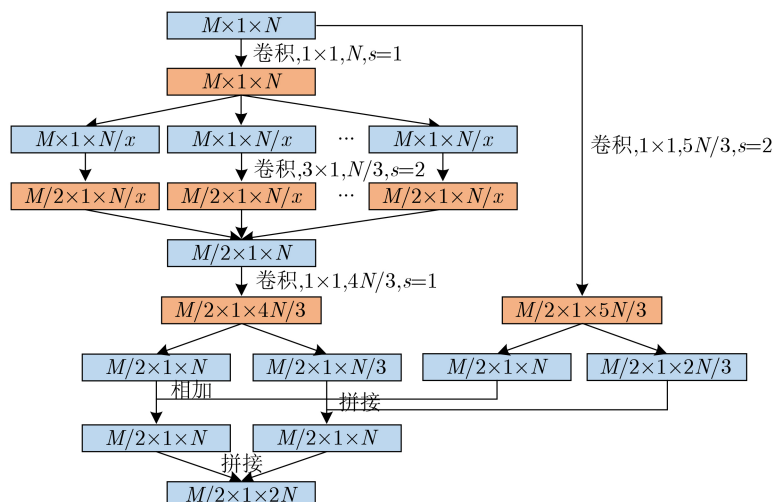
图3 卷积模块结构
