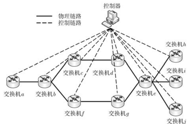
图 1 SDN 网络拓扑示意图
