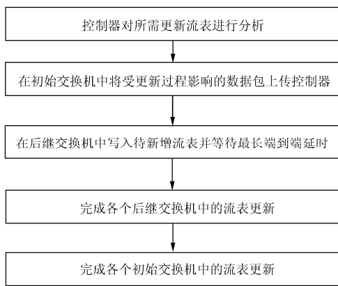
图2 基于一致性的SDN网络流表更新方案
