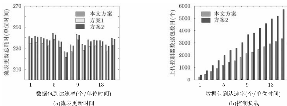
图5 单个初始交换机场景的仿真结果
