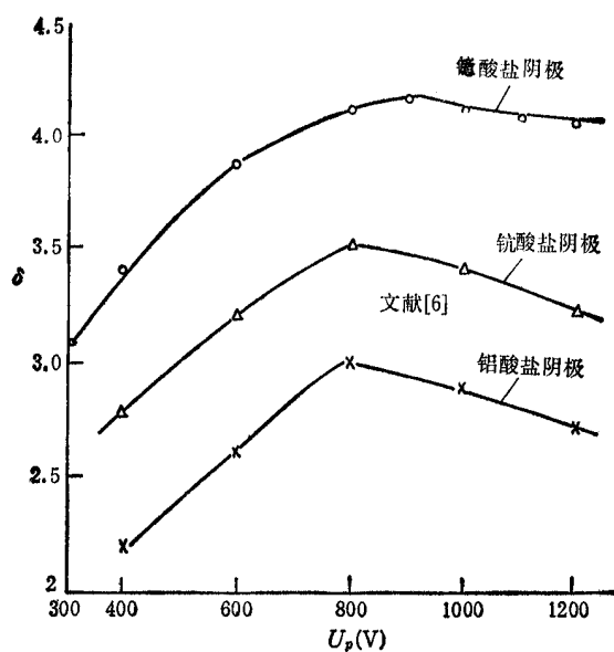
图4 阴极的次级发射系数与原电子电压的关 ( \delta-U_p )
