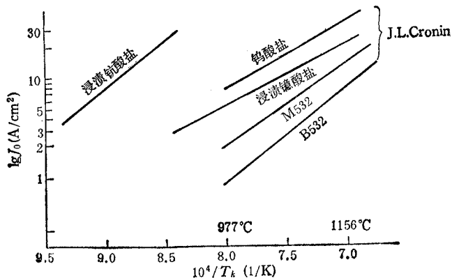
图 2 镱酸盐阴极, 钨酸盐阴极的 \lg J_{int} - T_K 曲线和国外报道的几种阴极的 \lg J_0 - T_K 曲线
