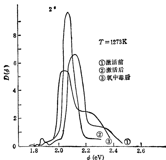
图3 钨酸盐阴极的逸出功分布
