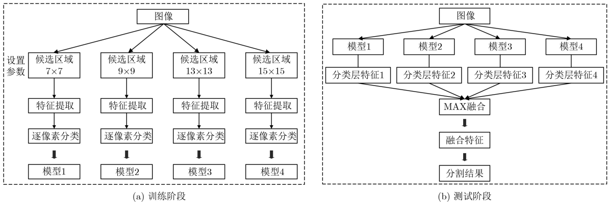
图4 模型融合框架示意图
