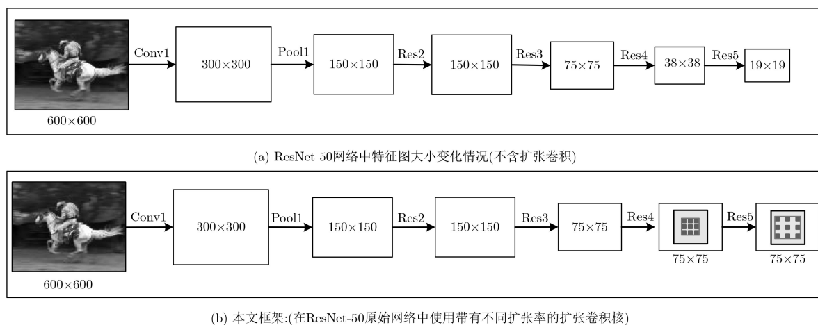
图2 带扩张卷积的卷积神经网络结构
