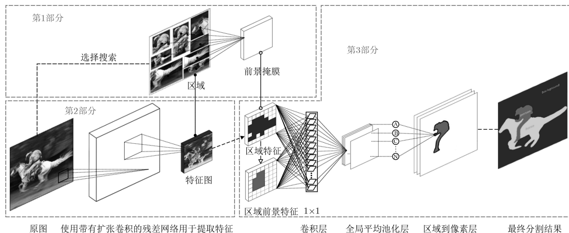
图1 本文所提模型框架
