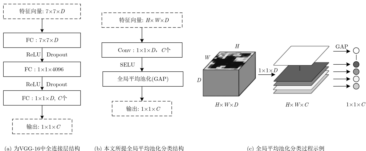
图3 全局平均池化层结构示意图
