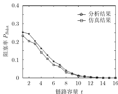
图7 网络 C(20,21,20, t )阻塞率随 t 变化图
