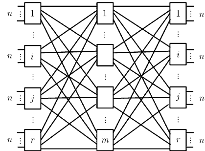
图1 三级 Clos 网络 C(n, m, r)
