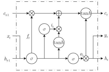
图1 长短期记忆网络单元结构
