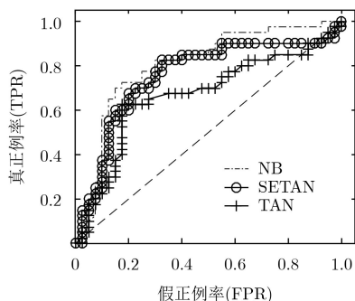
图5 二分类数据集的ROC曲线
