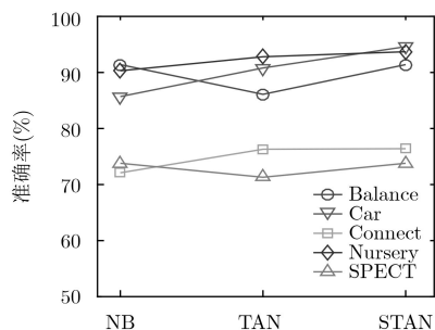
图4 平均分类准确率对比图
