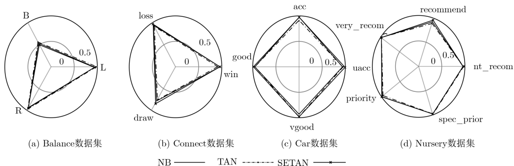
图 3 多分类数据集的AUC polar图对比
