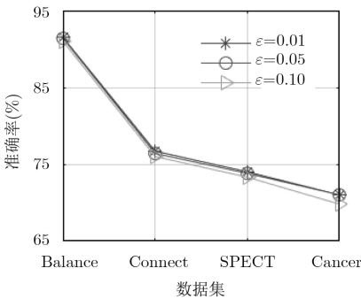
图 2 不同阈值 \varepsilon 的分类准确率
