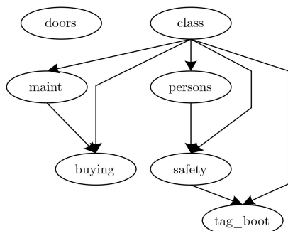
图7 SETAN结构示意图
