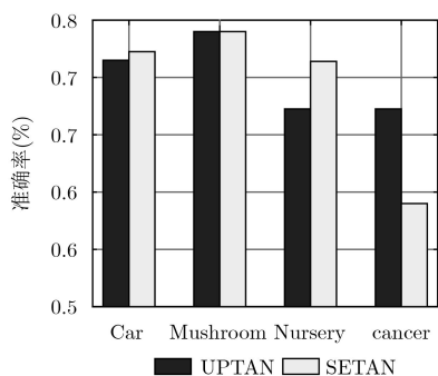
图6 平均分类准确率比较图
