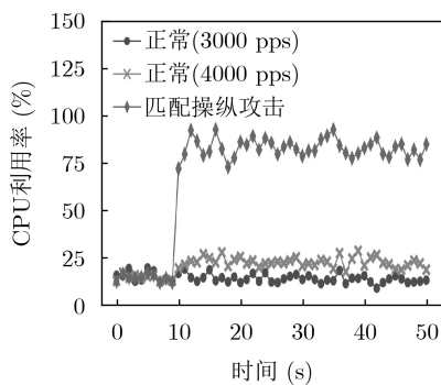
图7 匹配操纵攻击对控制器CPU的影响
